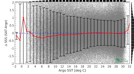
(b) Argo SST
