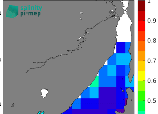
(d) Std(Argo SSS)
