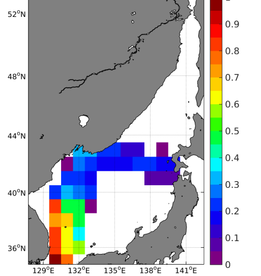
(d) STD(TSG-LEGOS-DM SSS)
