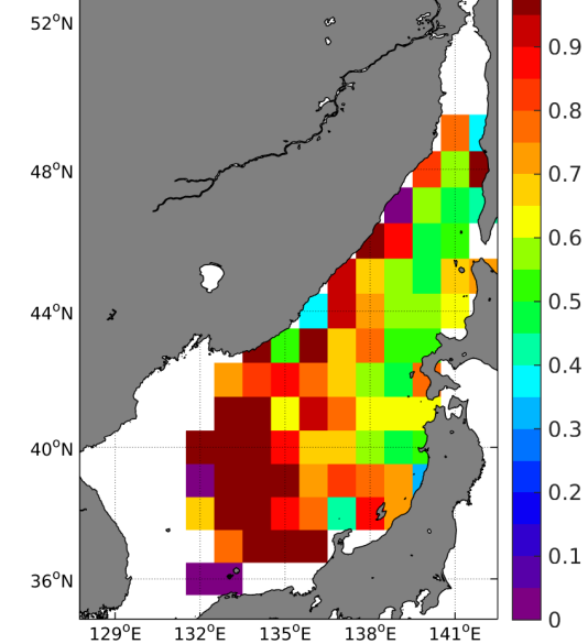
(b) STD(Satellite SSS)
