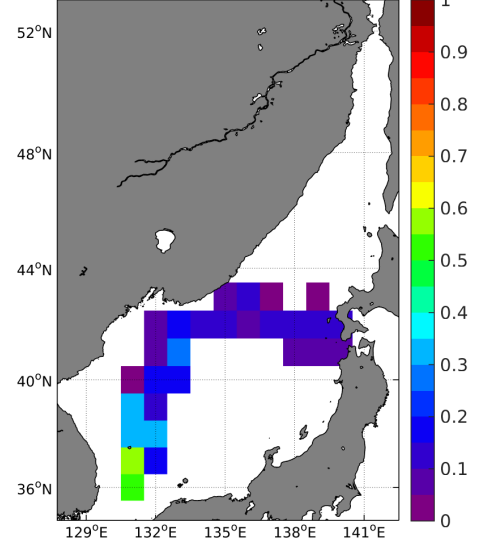
(d) STD(TSG-LEGOS-DM SSS)
