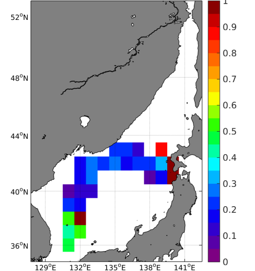
(f) STD( \Delta SSS) (Satellite - TSG-LEGOS-DM)
