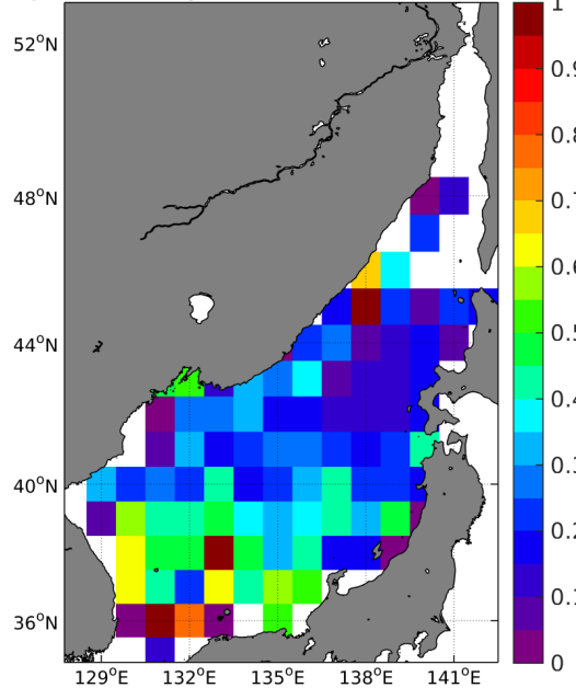
(d) STD(Argo SSS)
