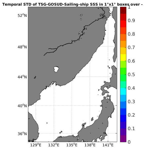
(d) STD(TSG-GOSUD-Sailing-ship SSS)
