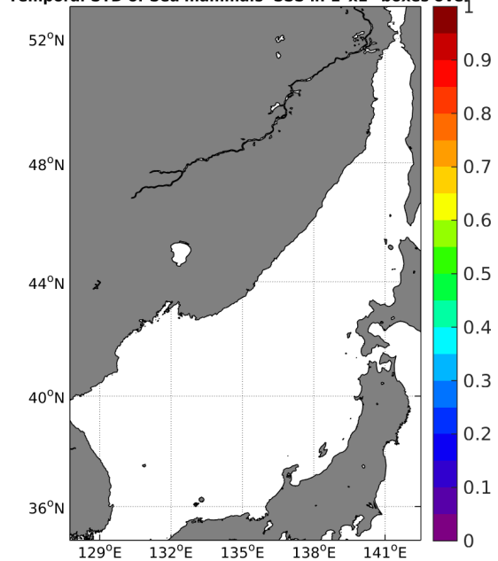
(d) STD(Sea mammals SSS)
