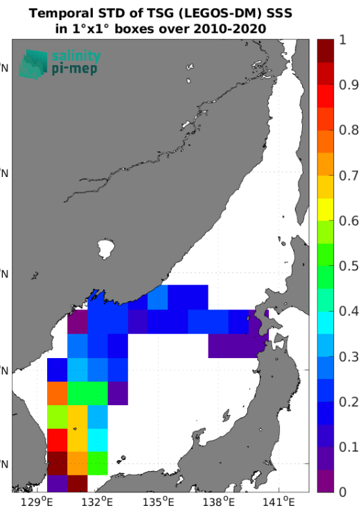
(d) Std(TSG (LEGOS-DM) SSS)
