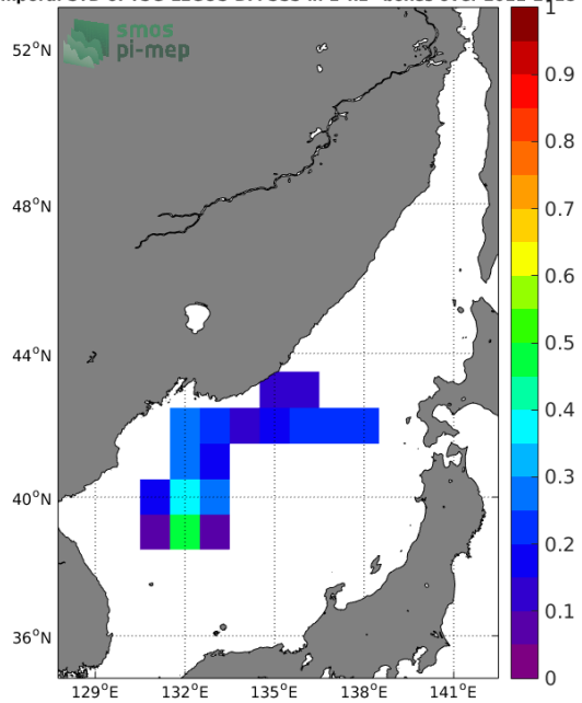
(d) STD(TSG-LEGOS-DM SSS)
