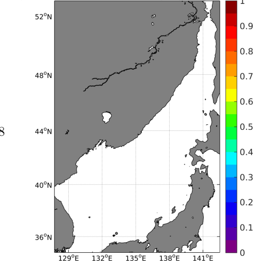
(f) STD(ΔSSS) (Satellite - TSG-GOSUD-Sailing-ship)
