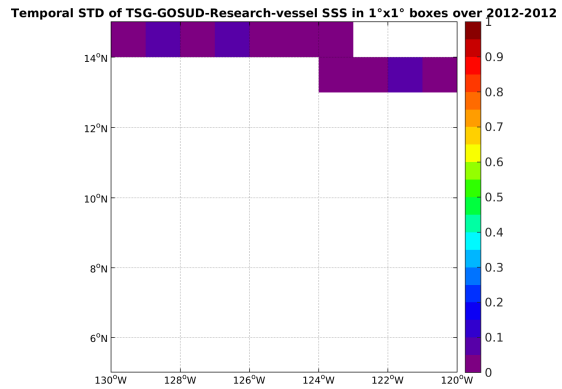
(d) STD(TSG-GOSUD-Research-vessel SSS)
