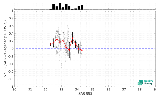
(b) ISAS SSS
