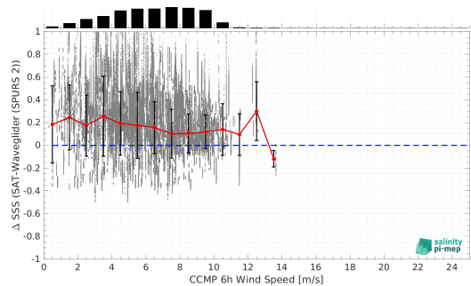
(d) CCMP Wind Speed
