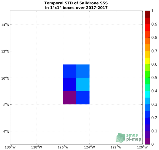
(d) Std(Saildrone SSS)
