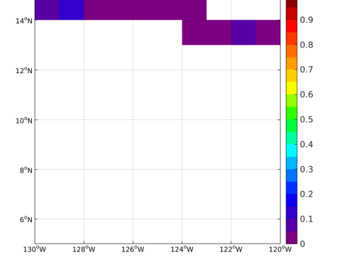
(d) STD(TSG-GOSUD-Research-vessel SSS)
