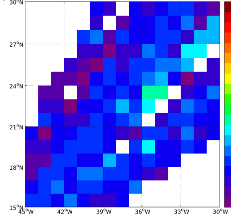
(f) STD( \Delta SSS) (Satellite - TSG-LEGOS-DM)
