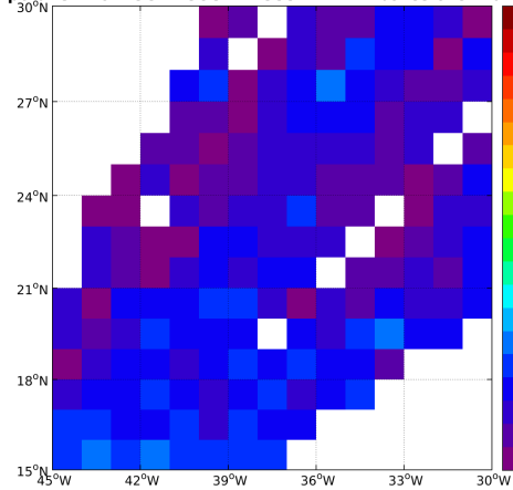
(d) STD(TSG-LEGOS-DM SSS)
