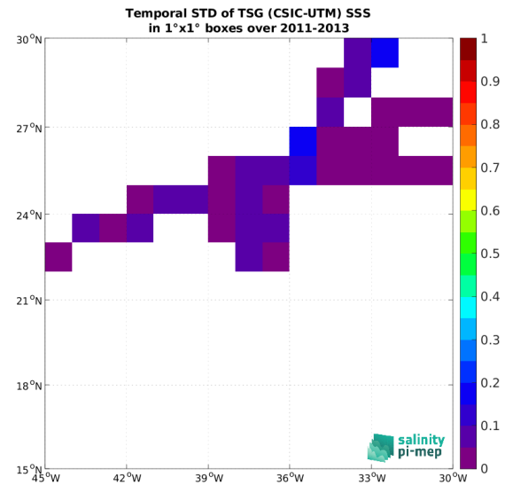
(d) Std(TSG (CSIC-UTM) SSS)
