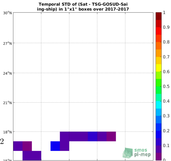
(f) Std( \Delta SSS) (Satellite - TSG-GOSUD-Sailing-ship)
