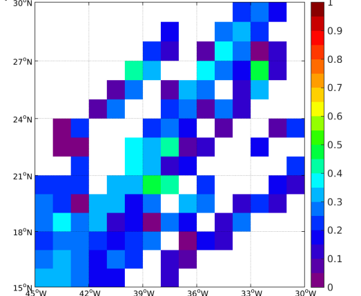
(f) STD( \Delta SSS) (Satellite - TSG-LEGOS-DM)
