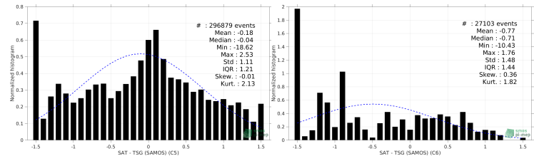
(d) WOA2013 SSS Std < 0.2 (e) WOA2013 SSS Std > 0.2
