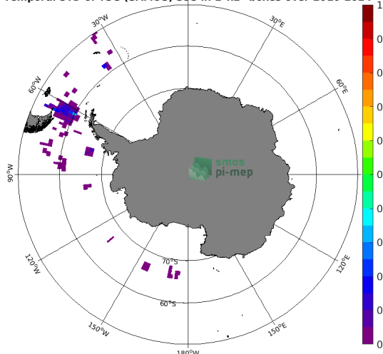
(d) Std(TSG (SAMOS) SSS)
