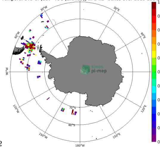
(f) Std( \Delta SSS) (Satellite - TSG (SAMOS))
