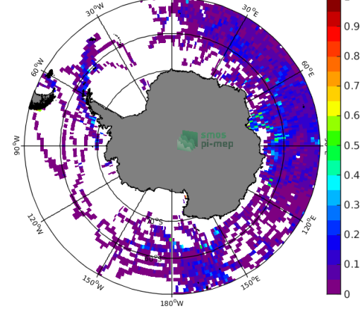
(d) Std(Sea mammals SSS)
