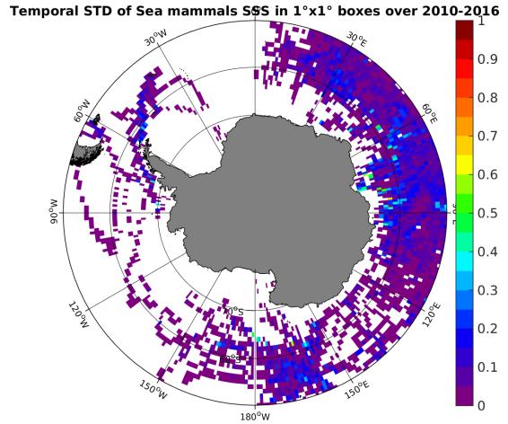
(d) STD(Sea mammals SSS)
