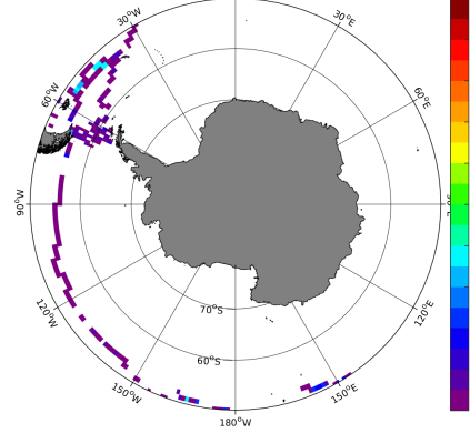
(d) STD(TSG-GOSUD-Sailing-ship SSS)
