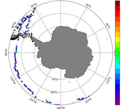
(f) STD( \Delta SSS) (Satellite - TSG-GOSUD-Sailing-ship)
