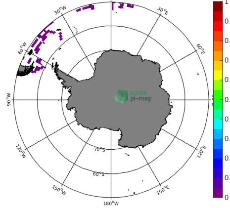
(d) Std(TSG-POLARSTERN SSS)
