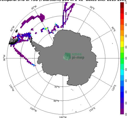
(d) Std(TSG (Polarstern) SSS)
