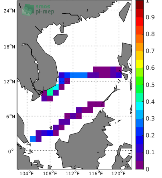
(d) Std(TSG-SAMOS SSS)
