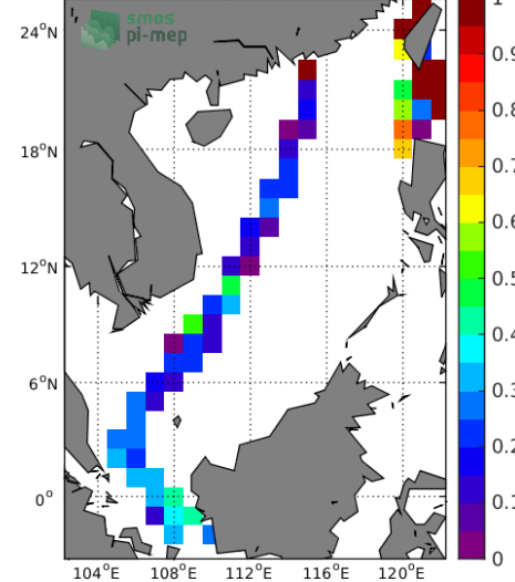
(f) Std( \Delta SSS) (Satellite - TSG-LEGOS-DM)
