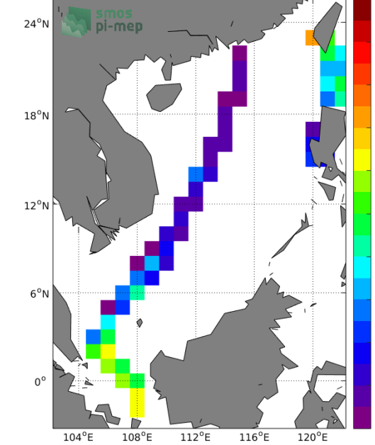
(d) Std(TSG-LEGOS-DM SSS)
