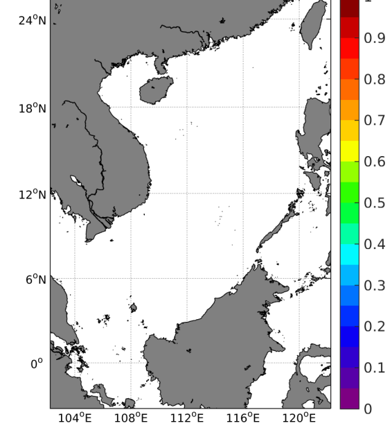
(d) STD(Sea mammals SSS)
