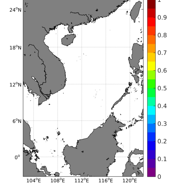
(d) STD(Surface drifters SSS)
