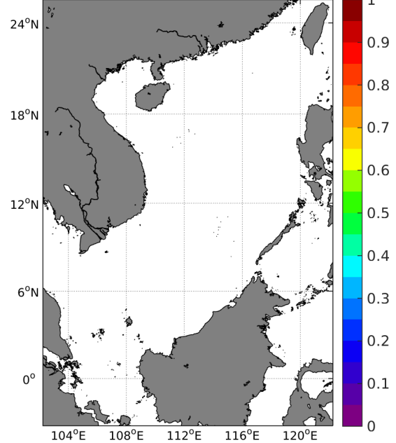
(d) STD(TSG-SAMOS SSS)
