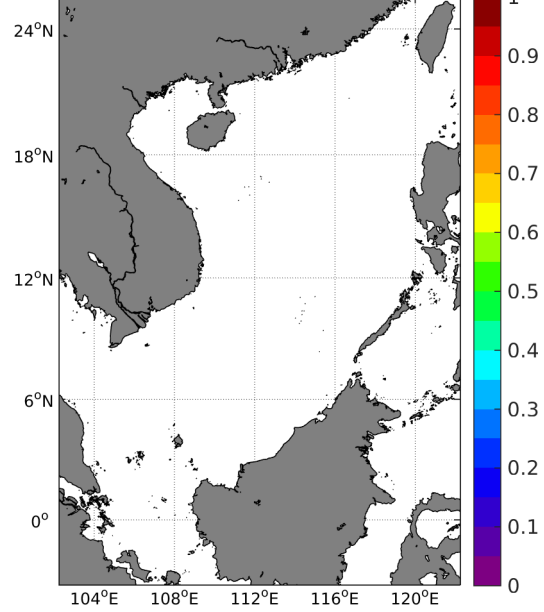
(d) STD(Surface drifters SSS)
