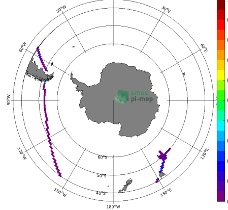
(d) Std(TSG (GOSUD-Research-vessel) SSS)
