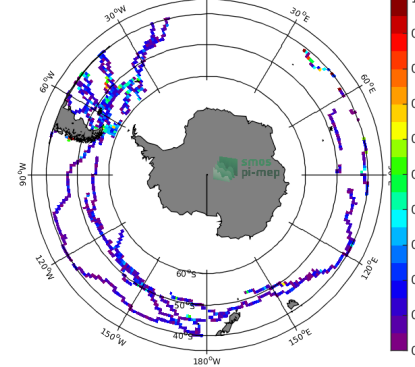
(f) Std( \Delta SSS) (Satellite - TSG-GOSUD-Sailing-ship)
