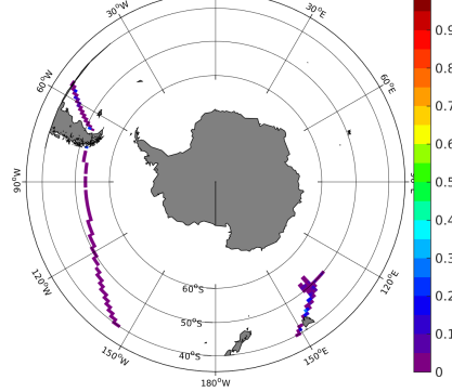
(d) STD(TSG-GOSUD-Research-vessel SSS)
