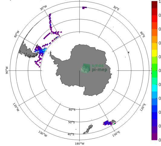
(f) Std( \Delta SSS) (Satellite - TSG (SAMOS))
