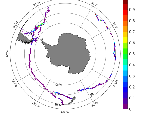
(f) STD( \Delta SSS) (Satellite - TSG-GOSUD-Sailing-ship)
