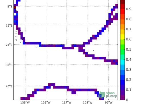
(f) Std( \Delta SSS) (Satellite - TSG-GOSUD-Sailing-ship)
