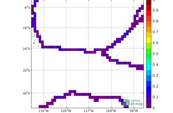
(f) Std( \Delta SSS) (Satellite - TSG-GOSUD-Sailing-ship)
