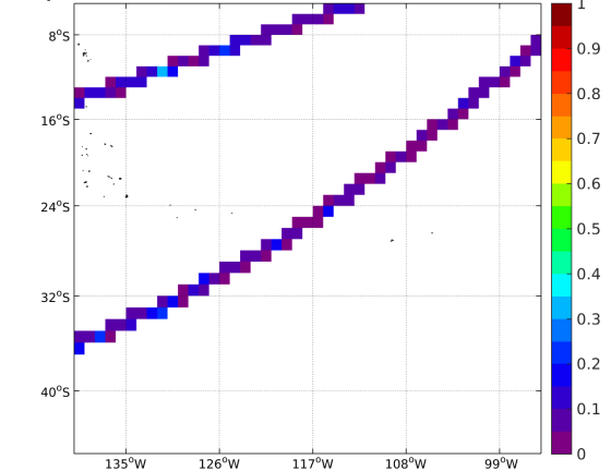
(f) STD( \Delta SSS) (Satellite - TSG-LEGOS-DM)
