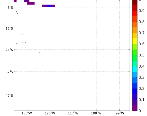
(d) STD(TSG-SAMOS SSS)
