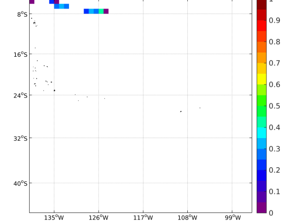
(f) STD( \Delta SSS) (Satellite - TSG-SAMOS)
