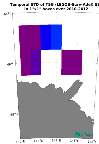
(d) Std(TSG (LEGOS-Surv-Adel) SSS)
