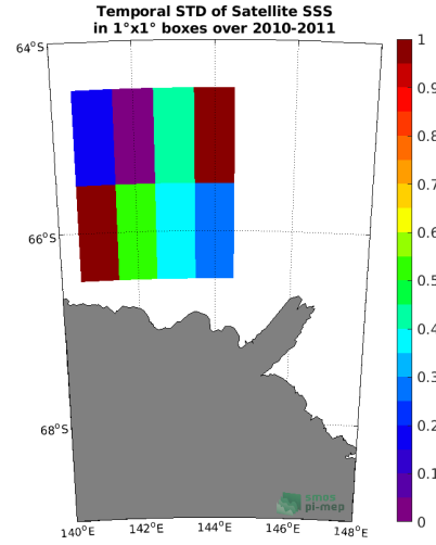
(b) Std(Satellite SSS)
