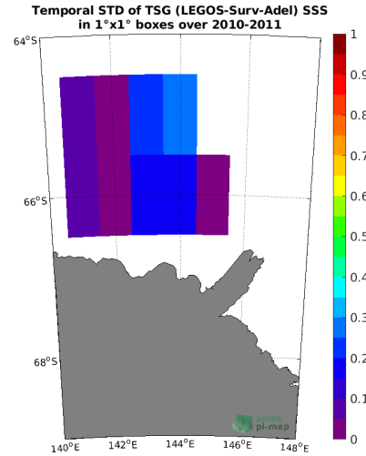
(d) Std(TSG (LEGOS-Surv-Adel) SSS)
