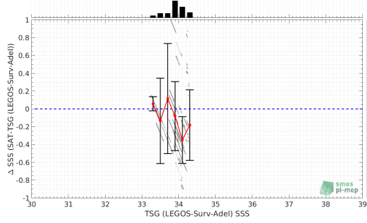
(a) TSG (LEGOS-Surv-Adel) SSS
