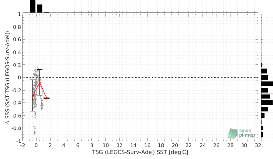
(b) TSG (LEGOS-Surv-Adel) SST
