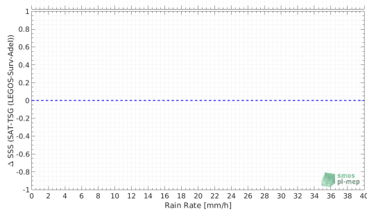
(d) CMORPH Rain rate
