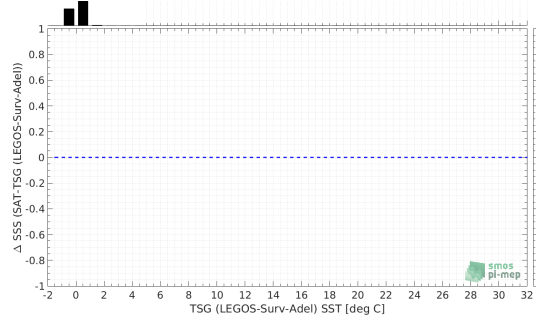
(b) TSG (LEGOS-Surv-Adel) SST
