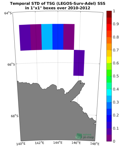
(d) Std(TSG (LEGOS-Surv-Adel) SSS)
