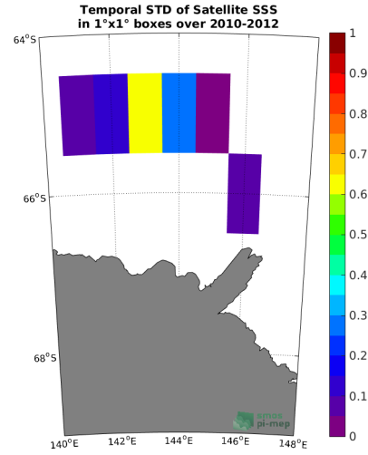
(b) Std(Satellite SSS)
