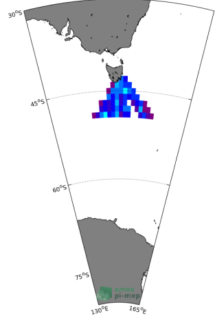
(b) STD(Satellite SSS)
