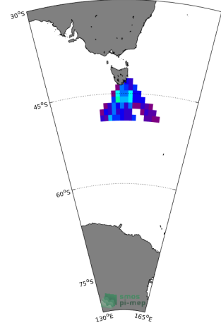
(d) STD(TSG-LEGOS-Survostral SSS)
