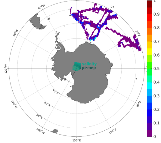
(d) Std(TSG (NCEI-0170743) SSS)
