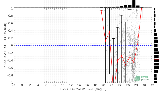
(b) TSG (LEGOS-DM) SST
